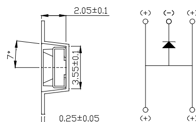
SEC:B-B'
